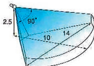
検知エリア図
